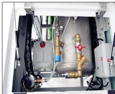
Wnętrze saturatora: zbiornik na wodę, lampa UV oraz zbiornik na wodę odciekową.
